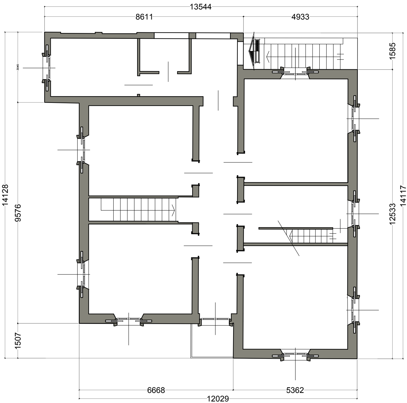
piano primo
